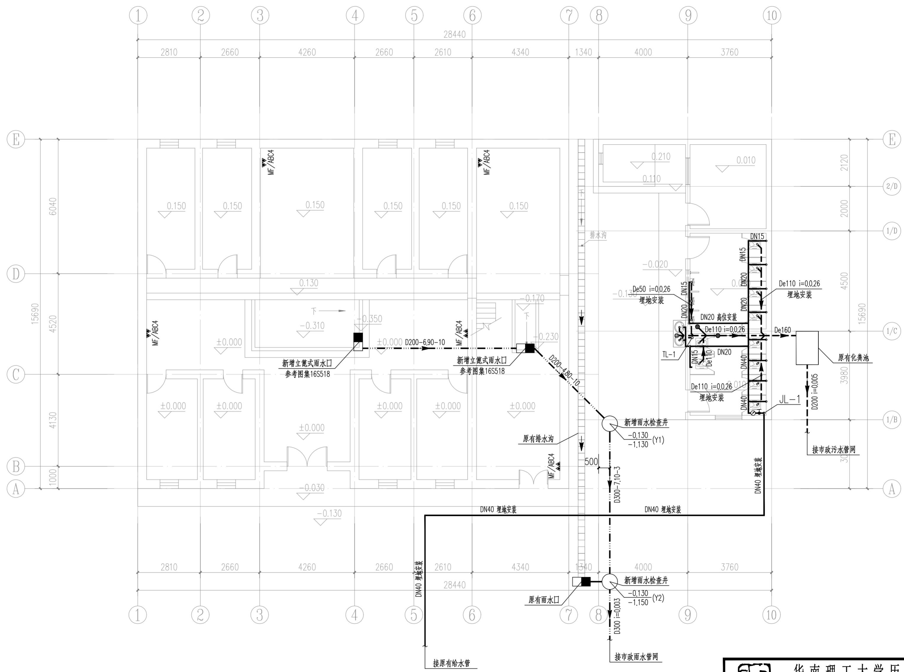
首层给排水平面图 1:100
